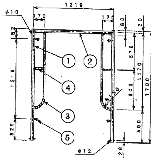
(構造図)
